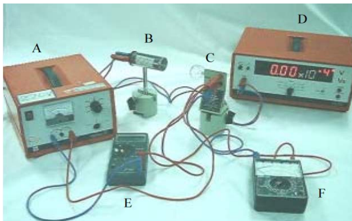
圖一：實驗儀器圖
