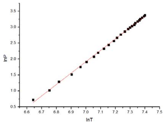
圖四:電功率與溫度的全對數圖
