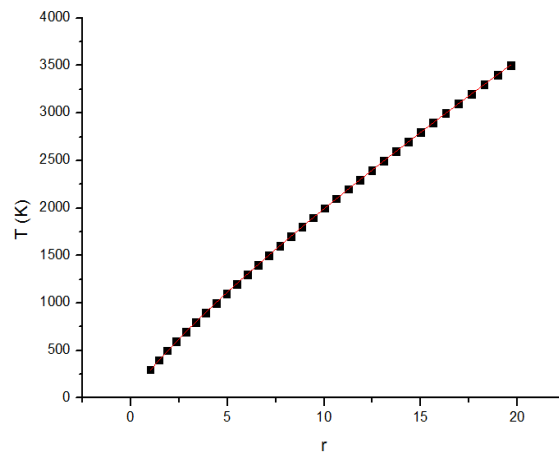
圖二: 電阻比值 r(=R/R_{300\text{K}}) 與溫度關係圖
